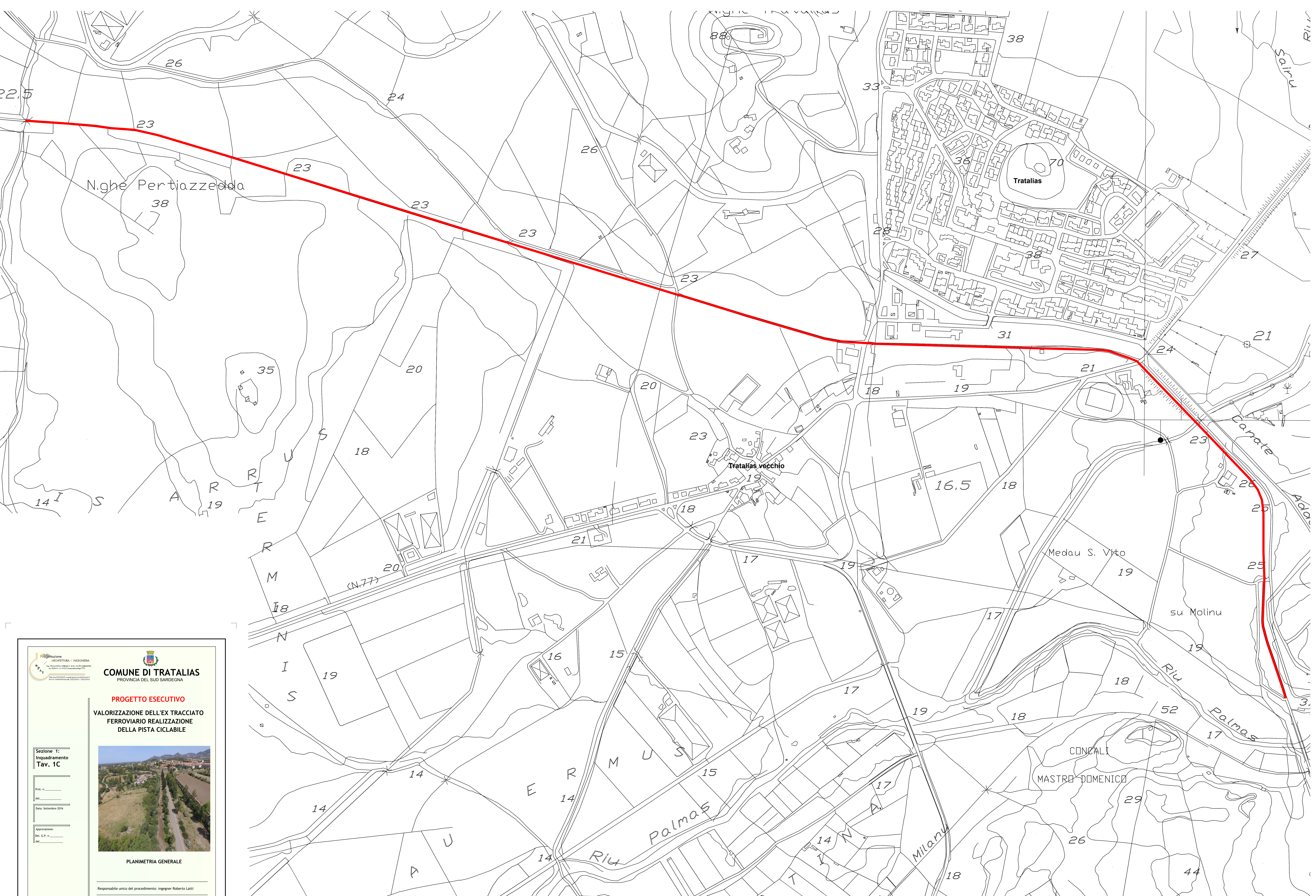
PLANIMETRIA GENERALE SCALA 1: 2500
